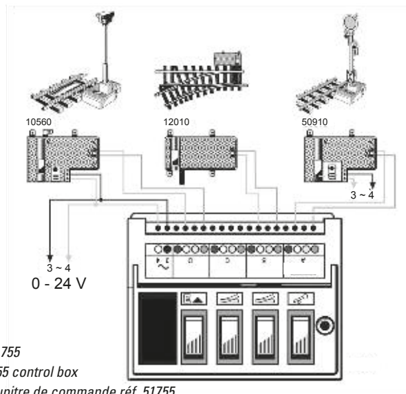
Afb. 3, Bedrijf met het bedieningskastje 51755
